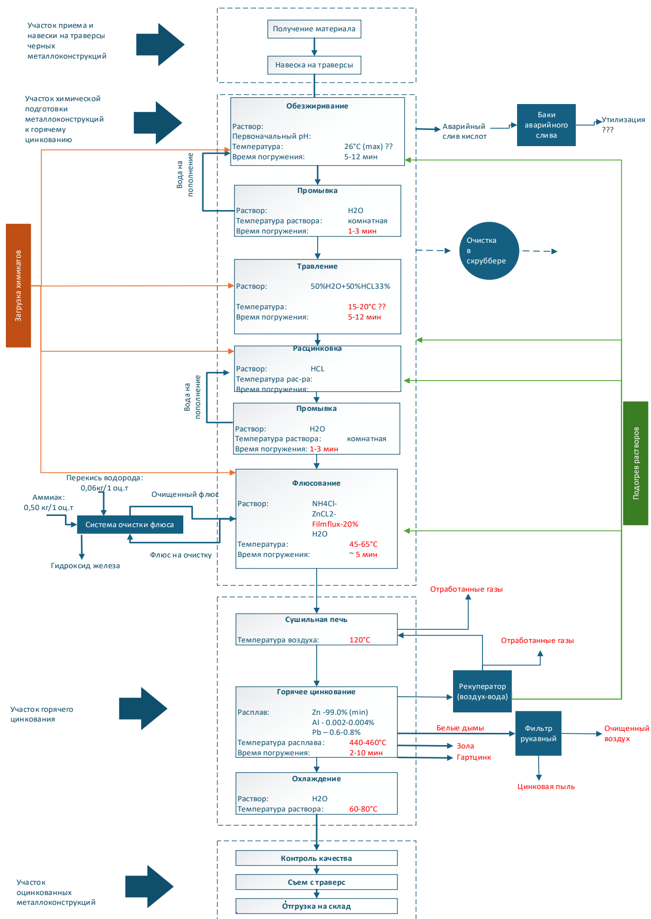
Рисунок 2.2 Блок-схема технологического процесса
