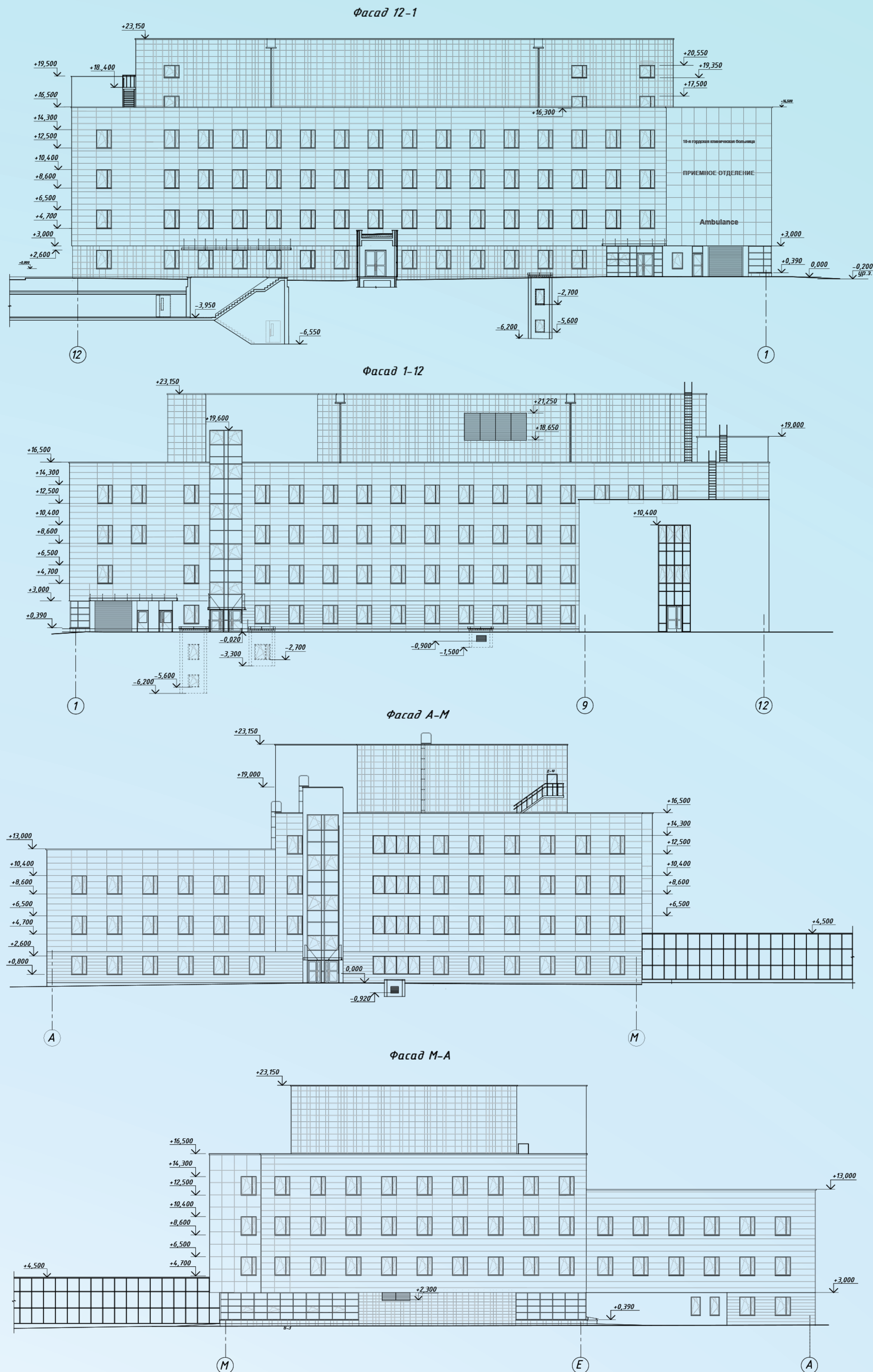
ФАСАДЫ ЗДАНИЯ
