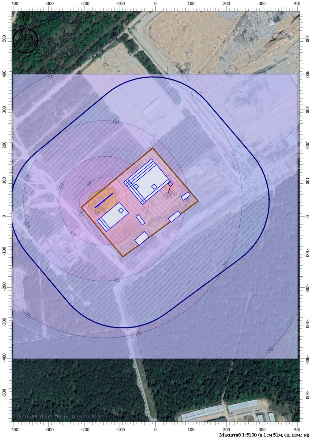
Рисунок Ж.1 – Рассеивание шума с учетом источников непостоянного шума
