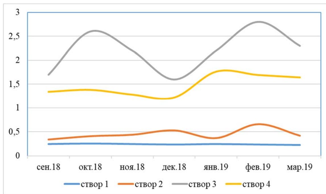
Рисунок 4.3 – Динамика изменения концентраций аммоний-иона в р. Свислочь ниже г. Минск в период с сентября 2018 г. по март 2019 г., мг/дм 3
